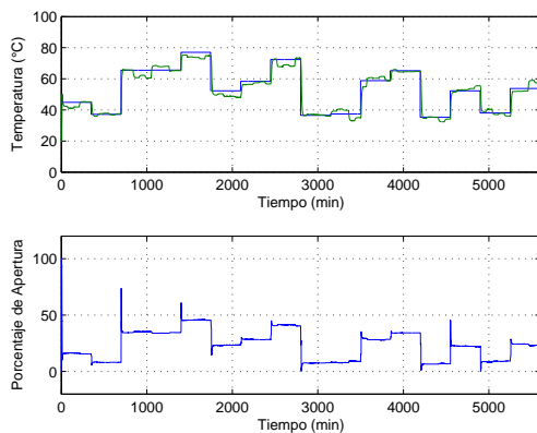
Figura 6. Resultados del controlador predictivo neuronal
