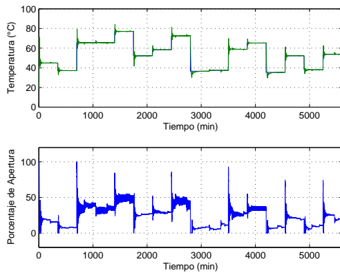
Figura 10. Resultados del controlador Feedforward
