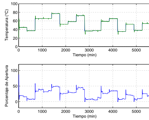
Figura 8. Resultados del controlador PID sintonizado por Algoritmos Genéticos
